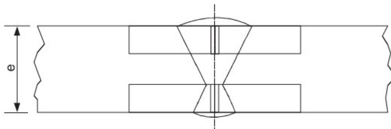
Suvirinimo siūlės vidurys
