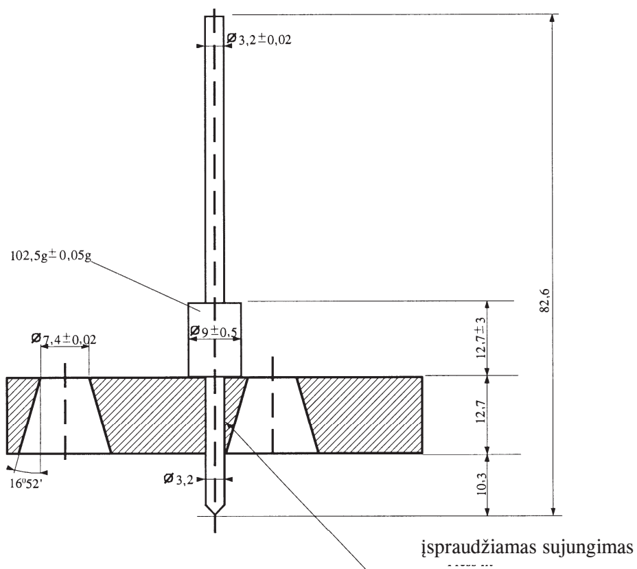
1 pav. Penetrometras
